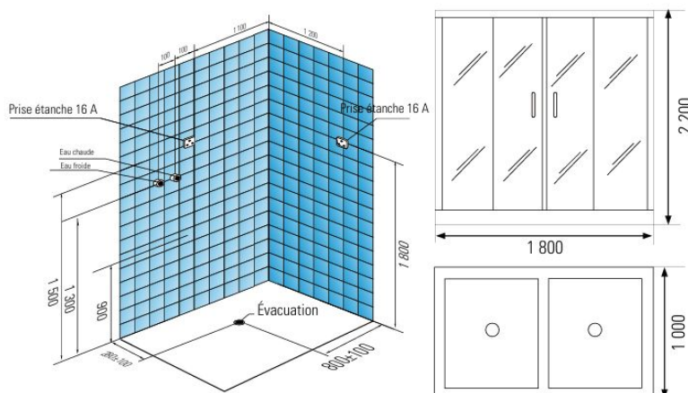
Schéma d'installation en 3D
